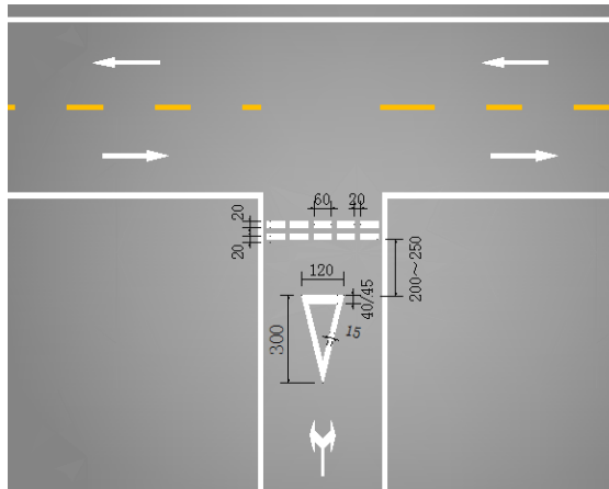
图 D.3 减速让标线 (单位: cm)
