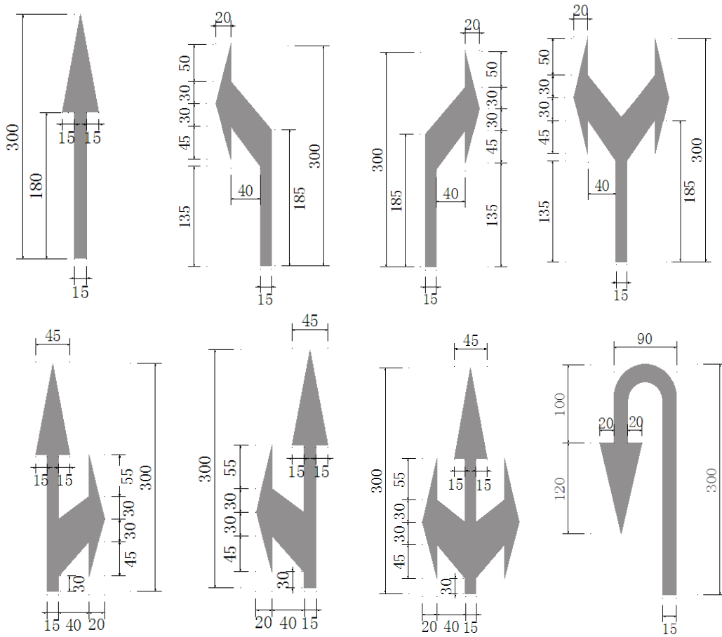
图 D.8 导向箭头 (单位: cm)
