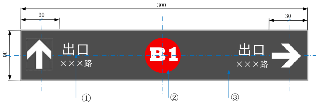
图 B. 10 车行出口引导标志牌示意及推荐尺寸（单位：cm）
