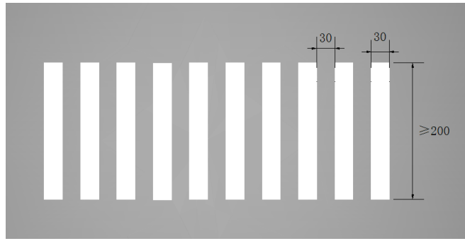
图 D.7 人行横道线 (单位: cm)
