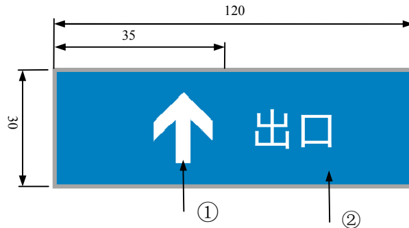
图 B. 11 车行出口引导标志牌示意及推荐尺寸（单位：cm）
