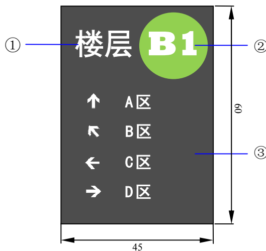
图 B. 19 楼层及区域指向标志牌示意及推荐尺寸 (单位: cm)
