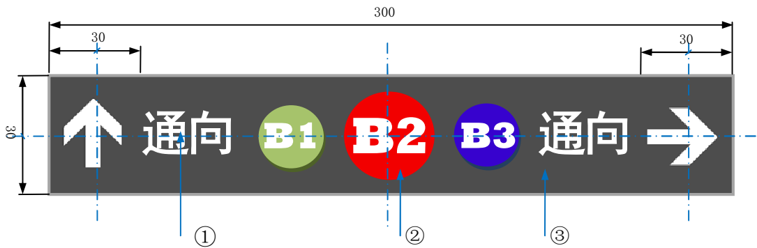
图 B. 16 停车楼层引导标志牌示意及推荐尺寸（单位：cm）
