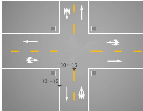
图 D.5 车行道边缘线（单位：cm）
