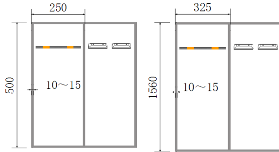
图 D. 9a) 垂直式停车位车位线 (单位: cm)
