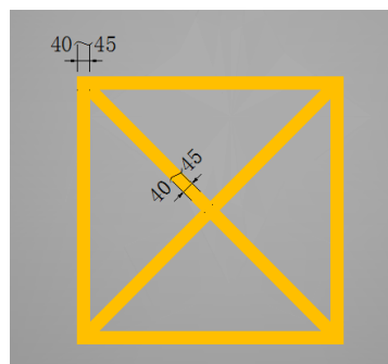
图 D.4 b) 简化网状线 (单位: cm)
