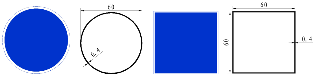
图 B.3 指示标志的底板及规格尺寸（单位：cm）
