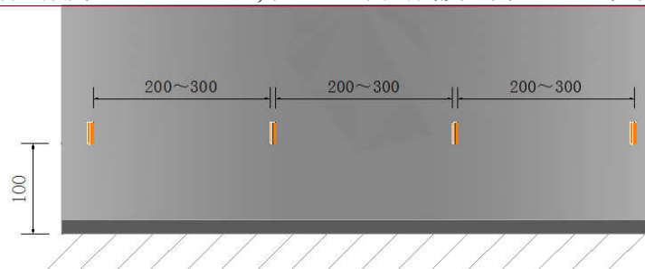
图 D. 13 轮廓标（单位：cm）
