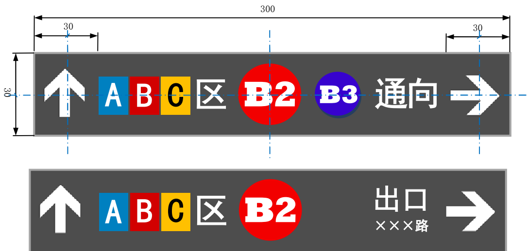
图 B. 17 组合引导标志牌示意及推荐尺寸（单位：cm）
