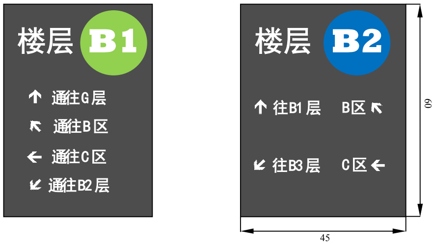
图 B. 20 停车楼层及区域指向标志牌示意及推荐尺寸（单位：cm）
