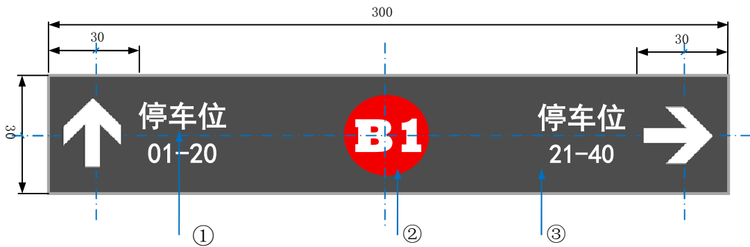
图 B. 13 停车位引导标志牌示意及推荐尺寸（单位：cm）
