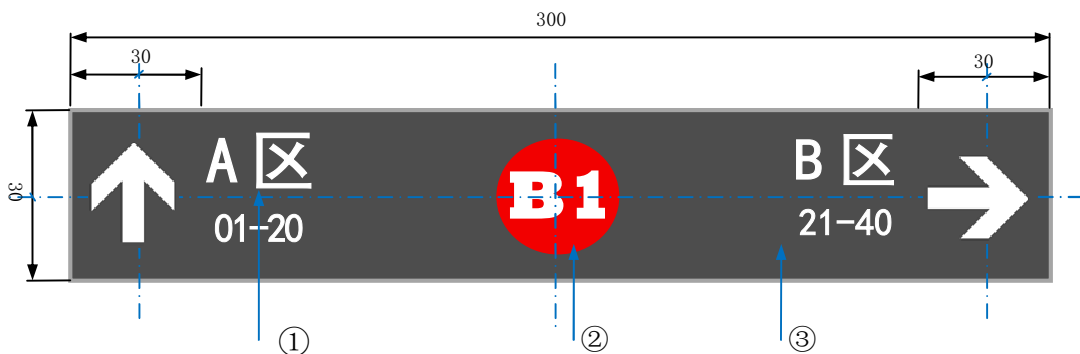
图 B. 12 停车区域引导标志示意及推荐尺寸（单位：cm）
