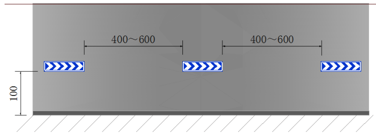
图 B. 22 线形诱导标 (单位: cm)
